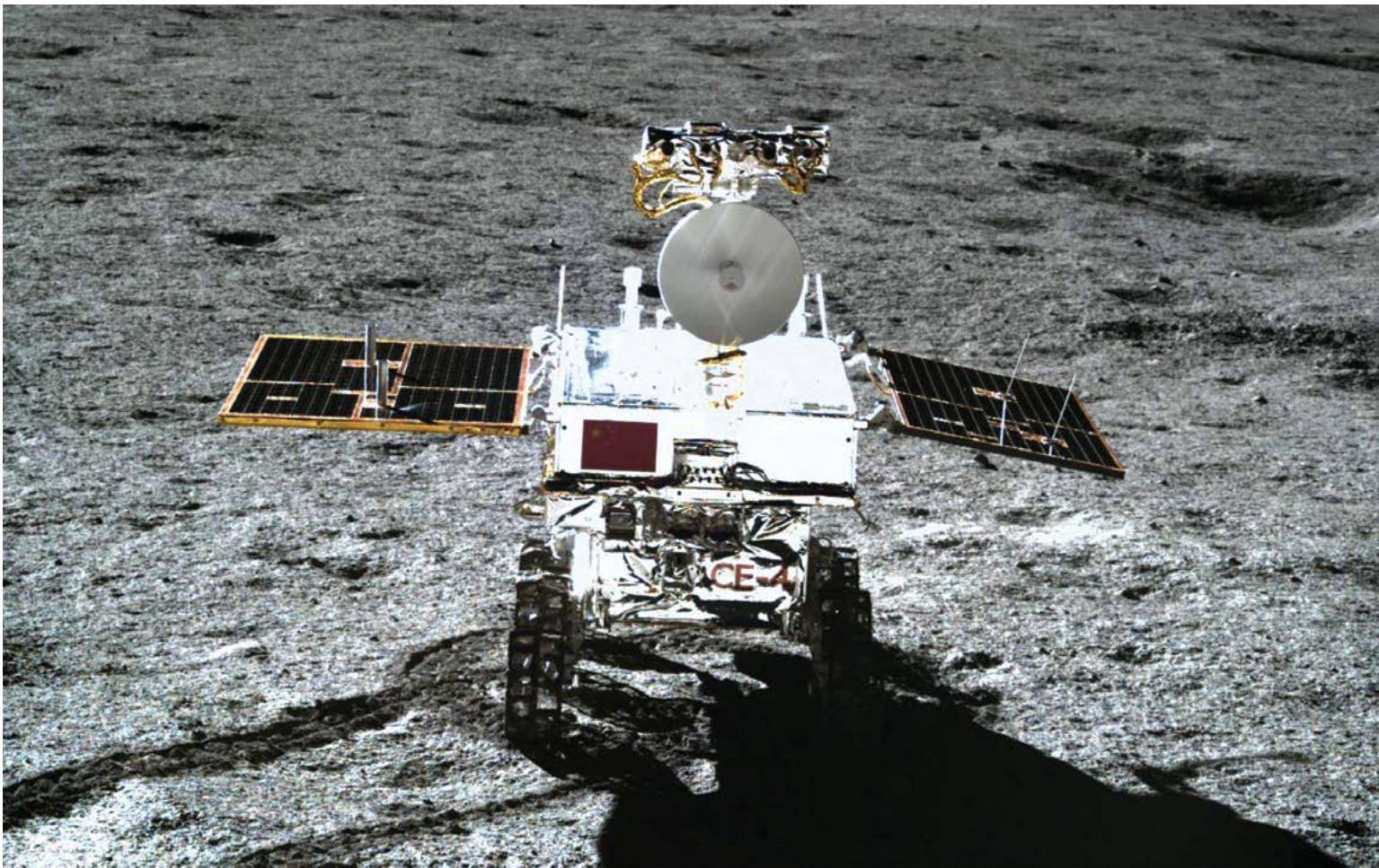
Phương tiện di chuyển trên mặt trăng, Yutu-2, được chụp bởi tàu thám dò mặt trăng Chang'e-4 ở phía xa của mặt trăng. Hình ảnh được công bố vào ngày 11/1/2019.
