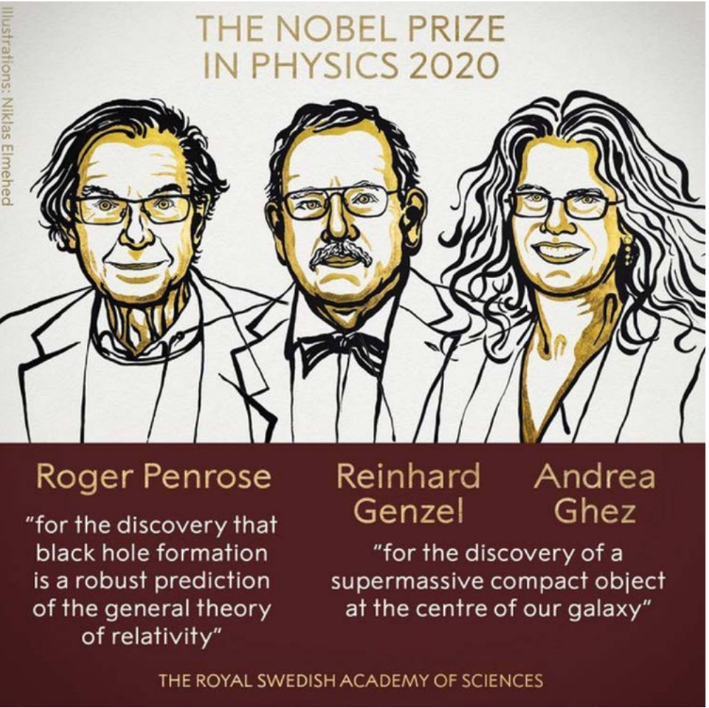
Các nhà khoa học được trao giải Nobel Vật lý 2020. Từ trái qua: Roger Penrose, Reinhard Genzel, Andrea Ghez.
