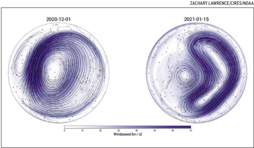
Trong khoảng thời gian từ tháng Mười Hai (trái) đến tháng Một (phải), xoáy cực đã di chuyển hoàn toàn khỏi Bắc Cực và cấu trúc đã bị thay đổi.
