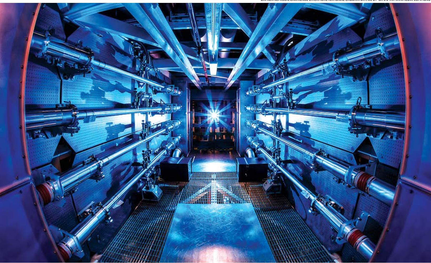
Bên trong cấu trúc hỗ trợ bộ tiền khuếch đại của Cơ sở Đánh lửa Quốc gia, giúp tăng năng lượng của chùm tia laser, tại Phòng thí nghiệm Quốc gia Lawrence Livermore ở Livermore, California, vào ngày 02/08/2012.
