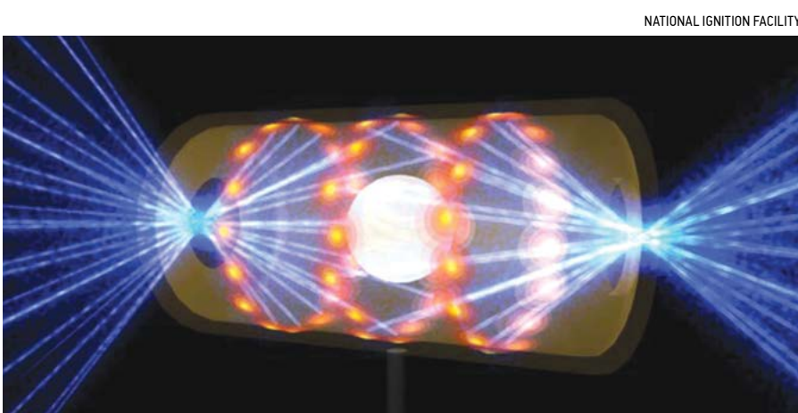
Mô hình diễn tả một viên đạn bị nhăm mục tiêu của NIF bên trong một khoang hốc (hohlraum) với các chùm tia laser đi qua các lỗ mở ở hai đầu. Các chùm tia này nén và đốt nóng mục tiêu đến các điều kiện cần thiết để xảy ra phản ứng nhiệt hạch.
