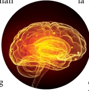
Giấc ngủ có vai trò quan trọng đối với một số chức năng của bộ não, bao gồm cách mà các tế bào thần kinh tương tác với nhau. SERGEY NIVENS/SHUTTERSTOCK
