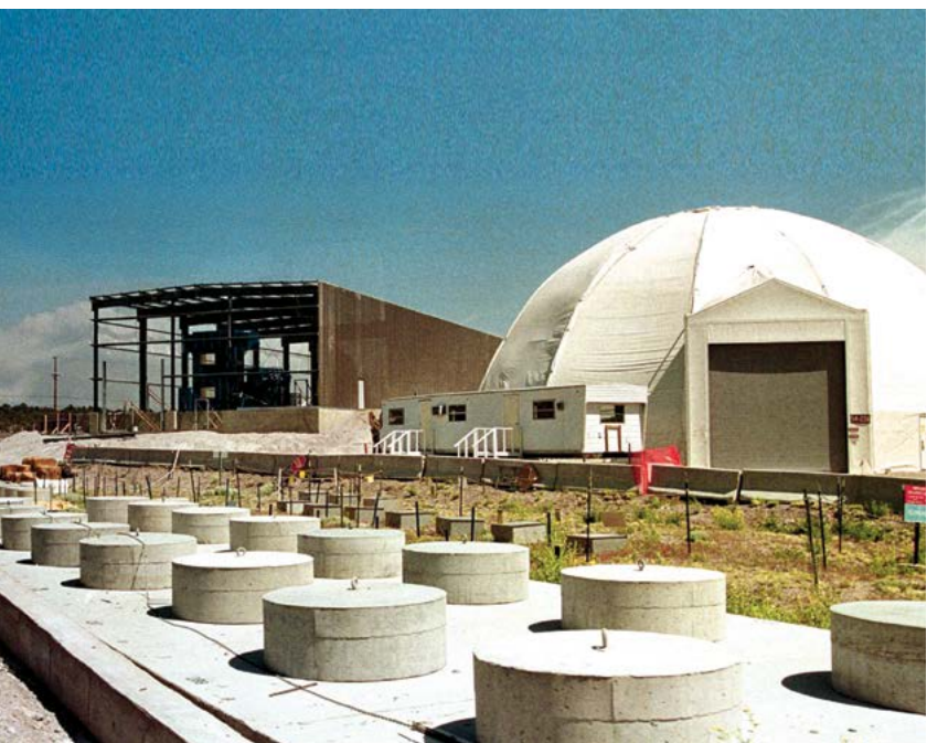
Nơi lưu trữ chất thải phóng xạ mức độ thấp tại Phòng thí nghiệm Quốc gia Los Alamos ở Los Alamos, New Mexico trong một bức ảnh tư liệu.
