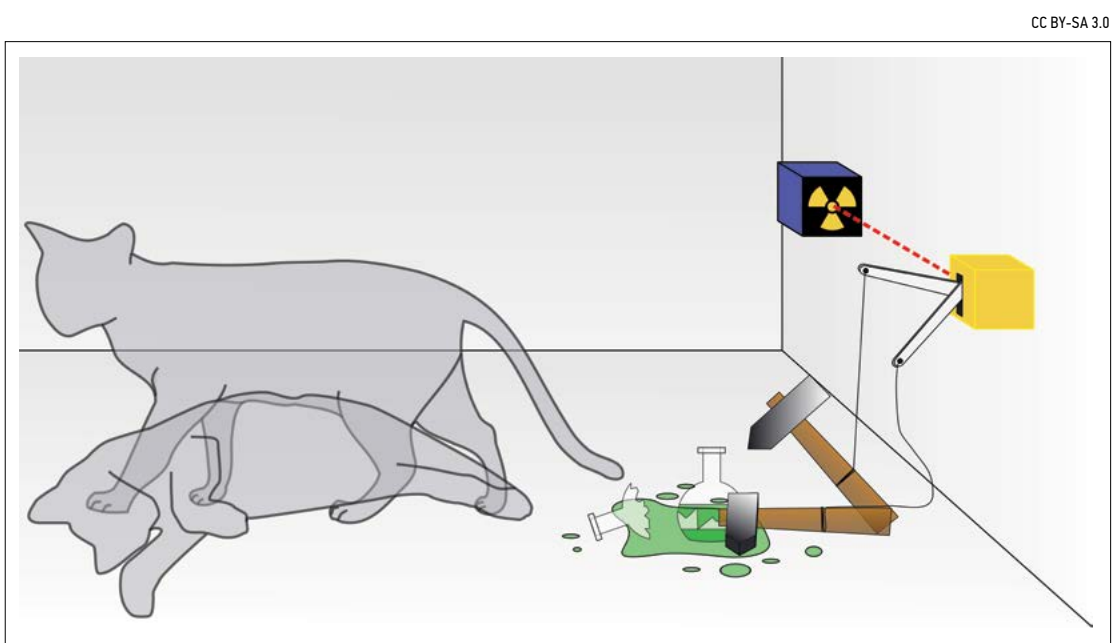
▲ Con mèo Schrodinger là một thí nghiệm tưởng tượng, và cũng là một trong những thí nghiệm nổi tiếng nhất trong cơ học lượng tử.
