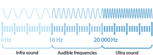
▲ Sóng hạ âm là sóng âm thanh có tần số dưới 20 hertz (Hz). Tần số sóng càng thấp, bước sóng càng lớn và càng khó che chắn.
